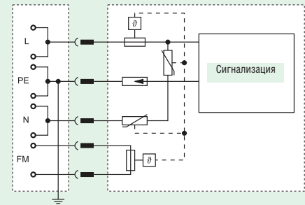
Схема соединения
