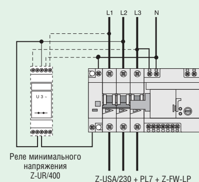
Схема соединения
