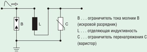
Принципиальная схема соединения
