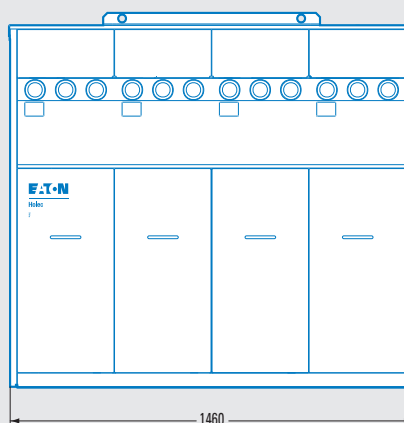
4-х секционная версия, вес 490 кг.
