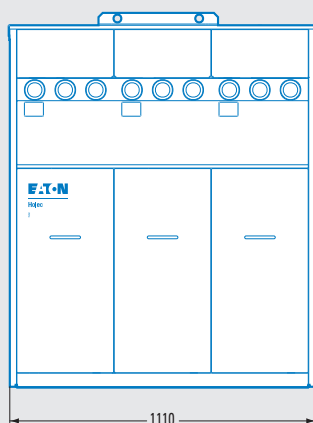
3-х секционная версия, вес 385 кг.
