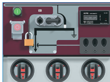
Заземленное положение.
